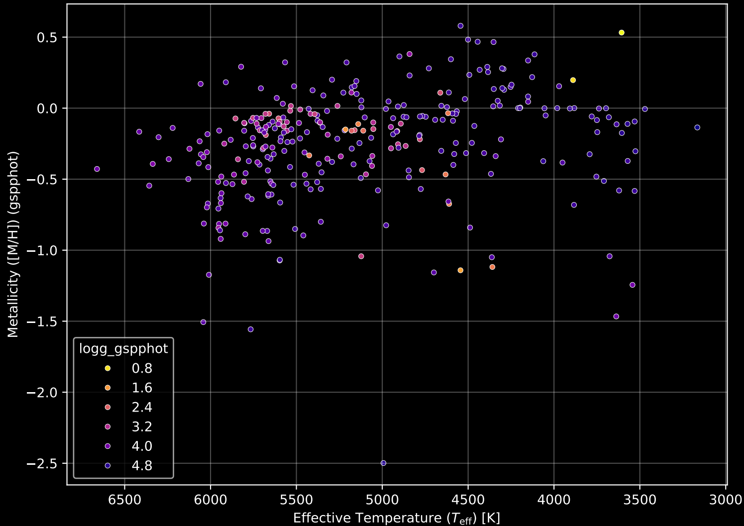
APOGEE DR17 Field: [N288] Stellar Population Parameters (n= 306)
